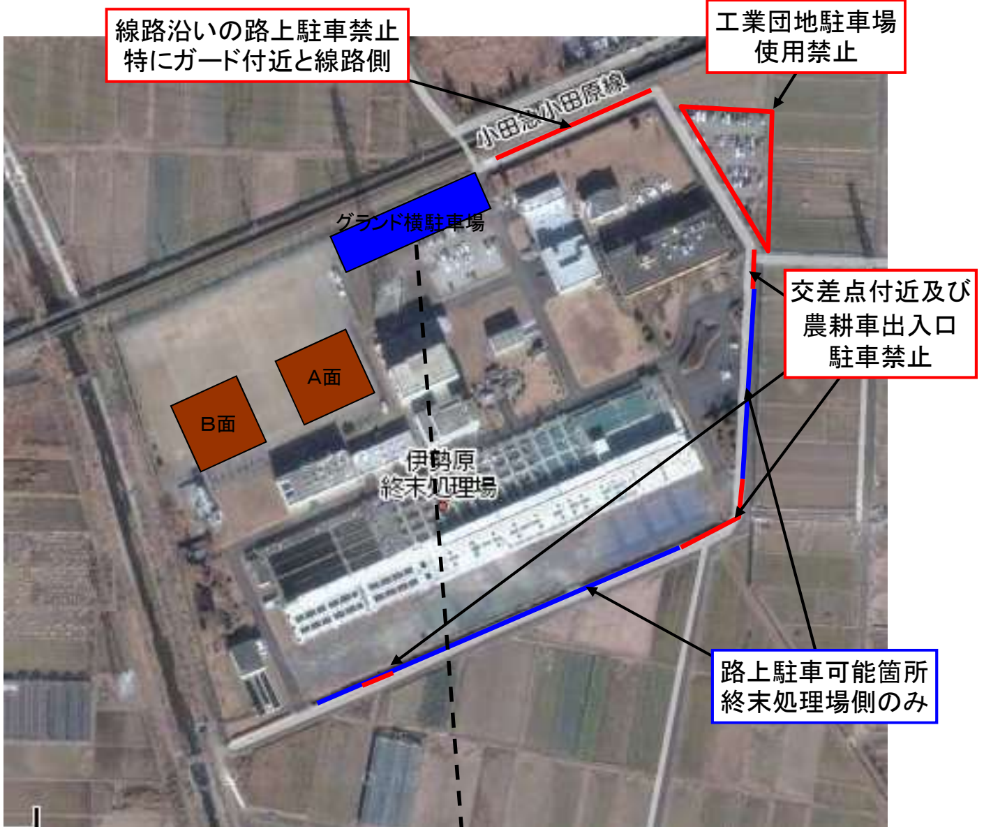
グランド横駐車場のレイアウト
