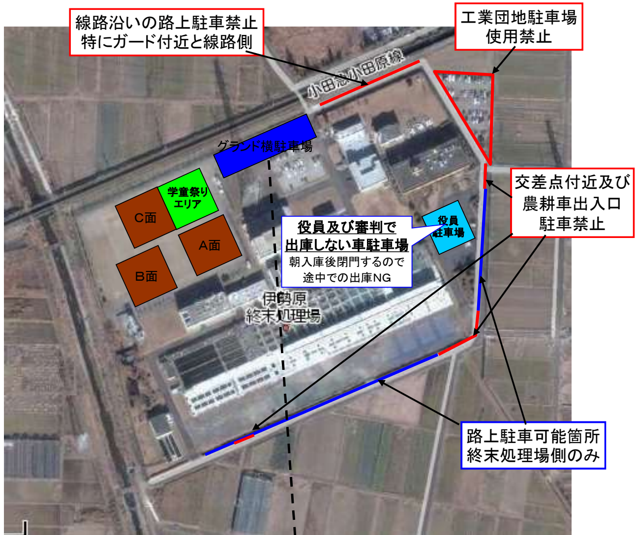
グランド横駐車場のレイアウト
